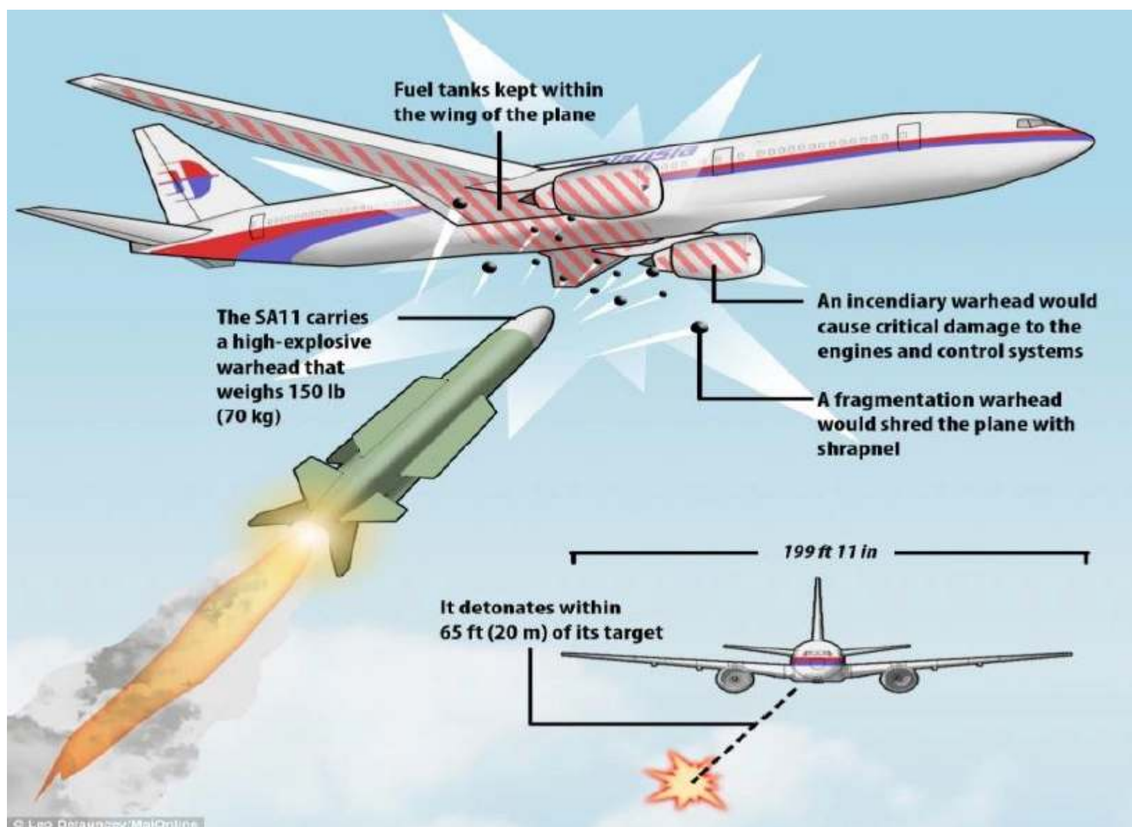
Buk raketos trajektorijos diagrama
